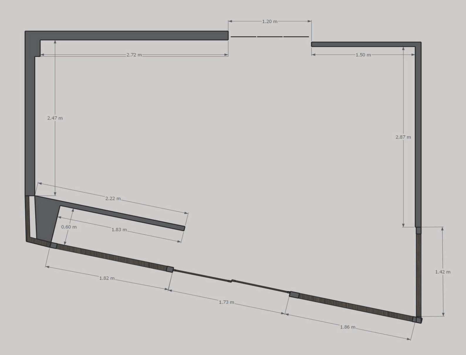
平面図
